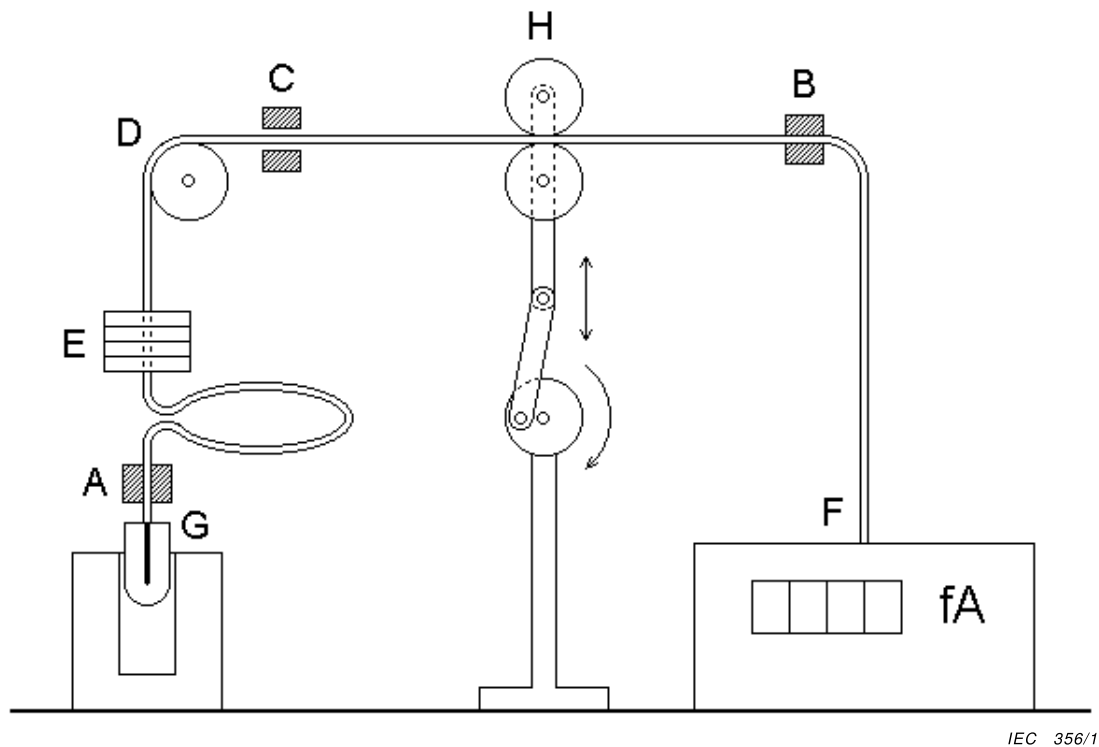
Figure B.1 – Appareillage d'essai pour la microphonie du câble
