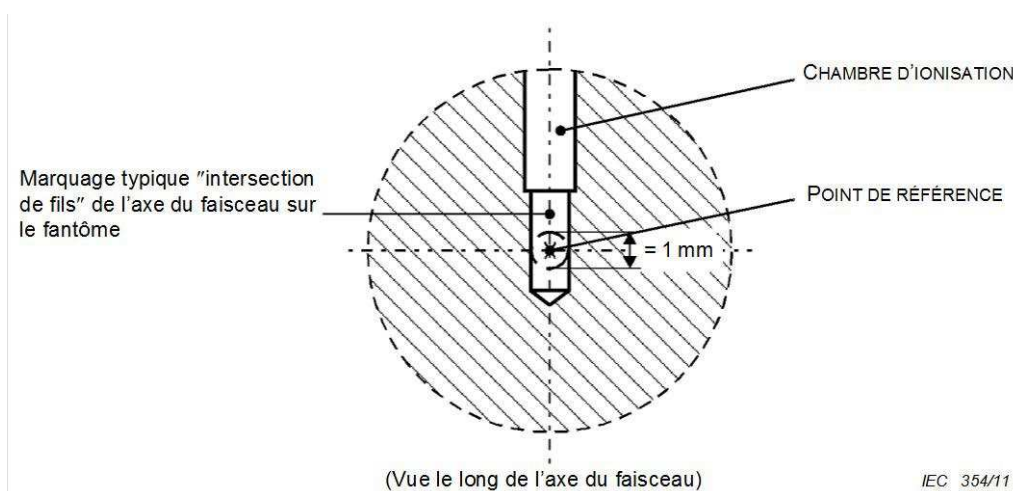
Figure 2 – Tolérance sur la position latérale dans le FANTÔME
